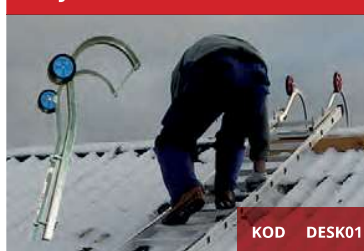
Specjalny element do mocowania drabiny na dachu. Special element used to fix the ladder on the roof.
